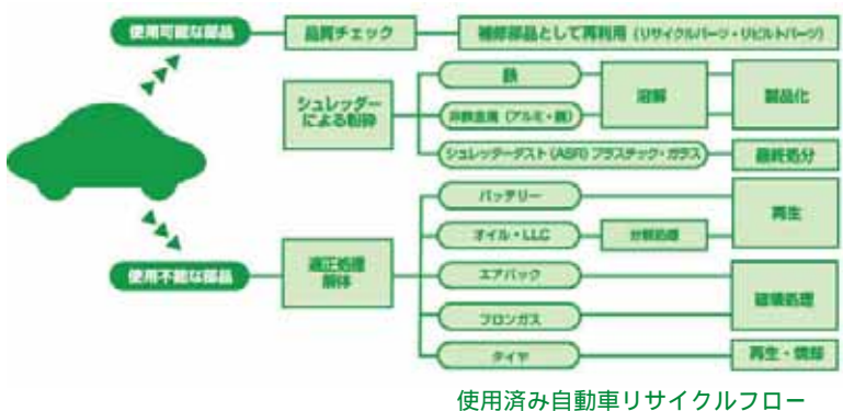
使用済み自動車リサイクルフロー
